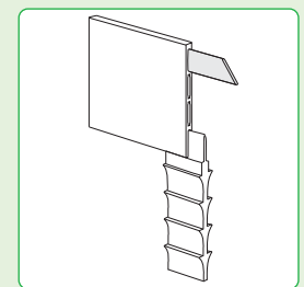
Profilé 200 mm avec ancre pour béton et jonction bout à bout
