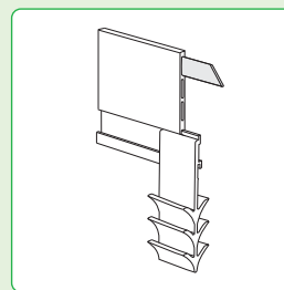
Profilé 120 mm avec ancre pour béton/tige d'ancrage et jonction bout à bout
