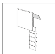
Profil 200 mm med beton-/jordanker og samlestykke
